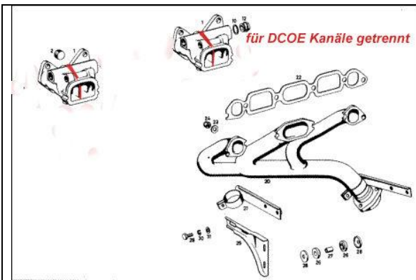
Ansaugkollektor für 2 x 40 DCOE Tubulures d'admission pour 2 40 DCOE
